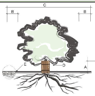
Ryc. 5. Zabezpieczenie pnia szalunkiem z desek (D), nawierzchnie antykompresyjne (E)
